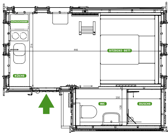
SKIZZE ERDGESCHOSS + DACHKAMMER
